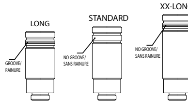
D. Piston Removal/Installation Désinstallation / Installation de piston
