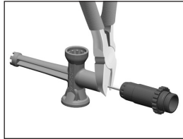
B. Nehmen Sie das Stabende ab
